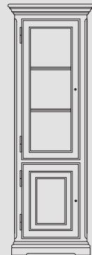
RU-358L Vitrine 1+1 trg. Türen links angeschlagen Innen: Oben 2 Holzfachböden, unten 1 Holzfachboden AD-120 Beleuchtungsset H/B/T: 190 x 62 x 45 RU-357L Schrank 1+1 trg. wie RU-358L jedoch obere Türe mit Holzfüllung
