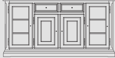
RU-356A Anrichte 4-trg. 2 Schub. li + re mit Glasfüllungen Innen: li+re je 2 Glasfachböden mittig 1 Holzfachboden H/B/T: 100 x 185 x 52 AD-127J Beleuchtungsset
