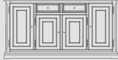
RU-356 Anrichte 4-trg. 2 Schub. Innen: li+re je 2 Holzfachböden mittig 1 Holzfachboden H/B/T: 100 x 185 x 52
