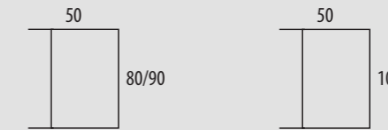
RU-168 Ansteckplatte 50 cm und doppelte Zargenkonstruktion (für Tischplattenbreite 80 und 90 cm), passend für Tisch RU-163 bis RU-167. Ab 110 cm Tischlänge möglich, extern zu lagern. Ab 115 cm Tischlänge sind 2 Ansteckplatte möglich, extern zu lagern. Zargenhöhe 8cm. Mittig keine Schublade möglich
